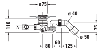
Siphon mit Bodenzulauf für Whirlwanne # 760451
