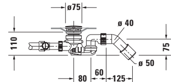
Siphon mit Bodenzulauf für Whirlwanne # 760450
