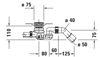
Siphon mit Bodenzulauf für Badewanne # 700451
