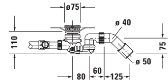
Siphon mit Bodenzulauf für Whirlwanne # 760449
