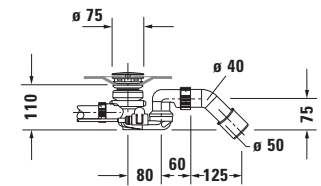
Siphon mit Bodenzulauf für Badewanne # 700449
