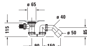
Siphon für Whirlwanne # 760451
