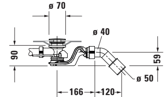
Siphon für Badewanne # 700450
