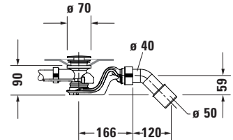
Siphon für Badewanne # 700451
