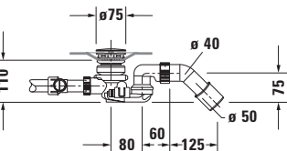
Siphon mit Bodenzulauf für Whirlwanne # 760453
