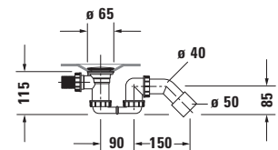
Siphon für Whirlwanne # 760449
