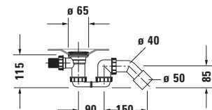
Siphon für Whirlwanne # 760450
